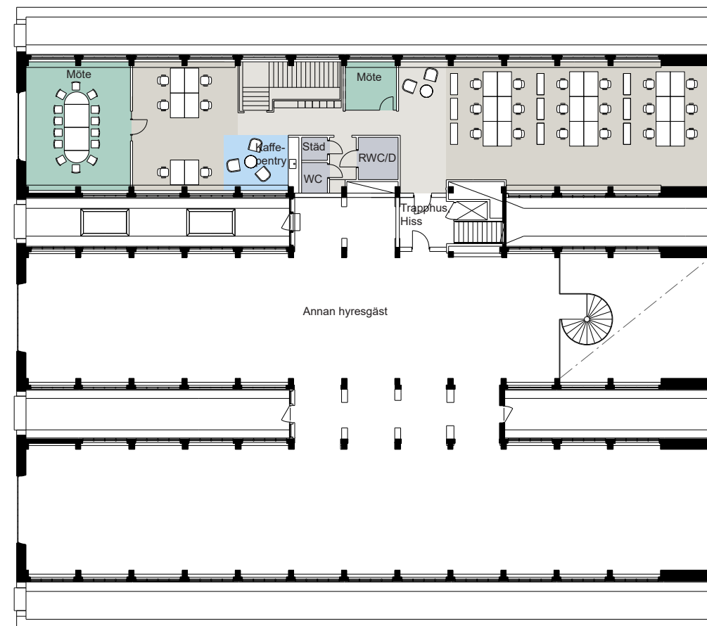
PLAN 1TR
